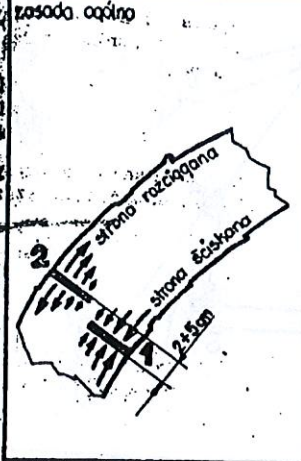
Kolejność i przesunięcie rzażów przy cięciu drewna
