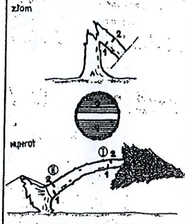
Kolejność i przesunięcie rzażów przy cięciu drewna
