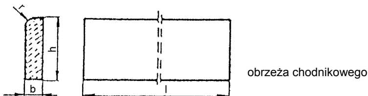
Rysunek 1. Kształt betonowego obrzeża chodnikowego Tabela 1. Wymiary obrzeży
