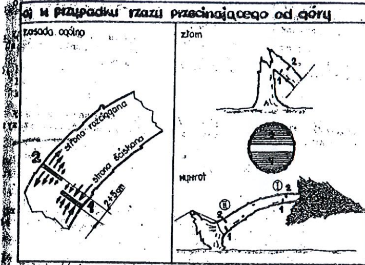
Kolejność i przesunięcie rzażów przy cięciu drewna
