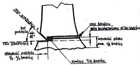
A. Podstawowe zasady wykonywania rzazów przy ścinie drzewa.
