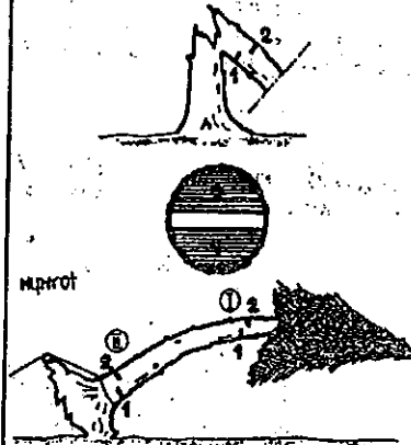
Kolejność i przesunięcie rzażów przy cięciu drewna
