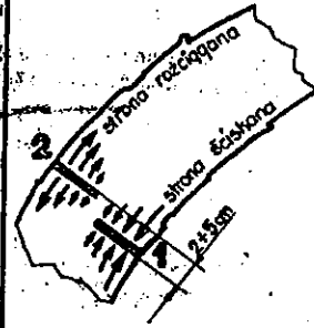
Kolejność i przesunięcie rzażów przy cięciu drewna
