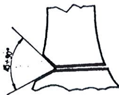
B. Wykonanie rzazu podcinającego dwoma cięciami ukośnymi. Rząd ścinający na poziomie zetknięcia się rzazów podcinających
