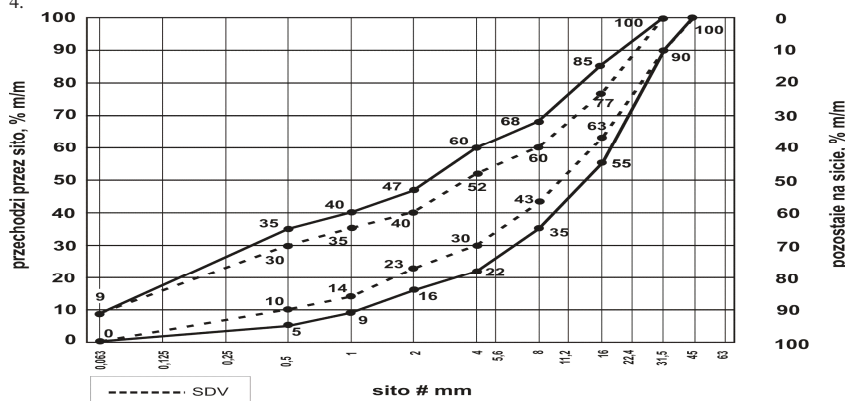
Rys. 3. Uziarnienie mieszanki niezwiązanej 0/31,5 dla podbudowy zasadniczej
