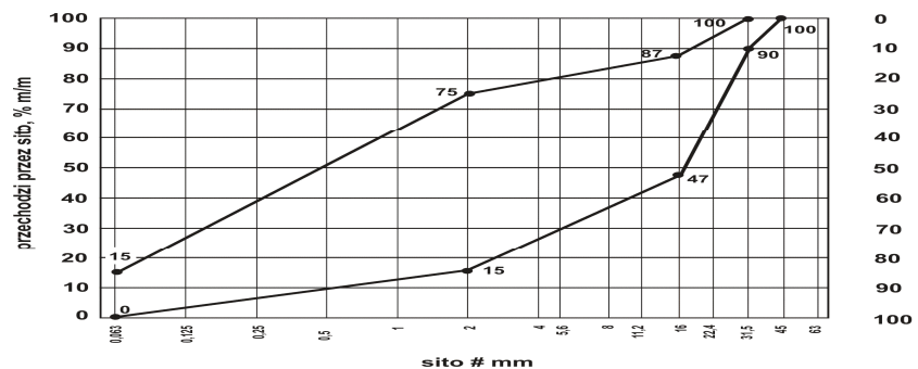
Rys. 4. Uziarnienie mieszanki niezwiązanej 0/31,5 dla nawierzchni
