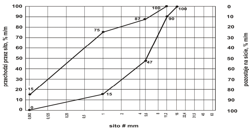
Rys.1. Uziarnienie mieszanki niezwiązanej 0/11,2 dla warstwy mroзоochronnej
